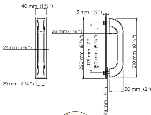
B16.BHGLMP Paire de poignées de bain Glasgow métal
